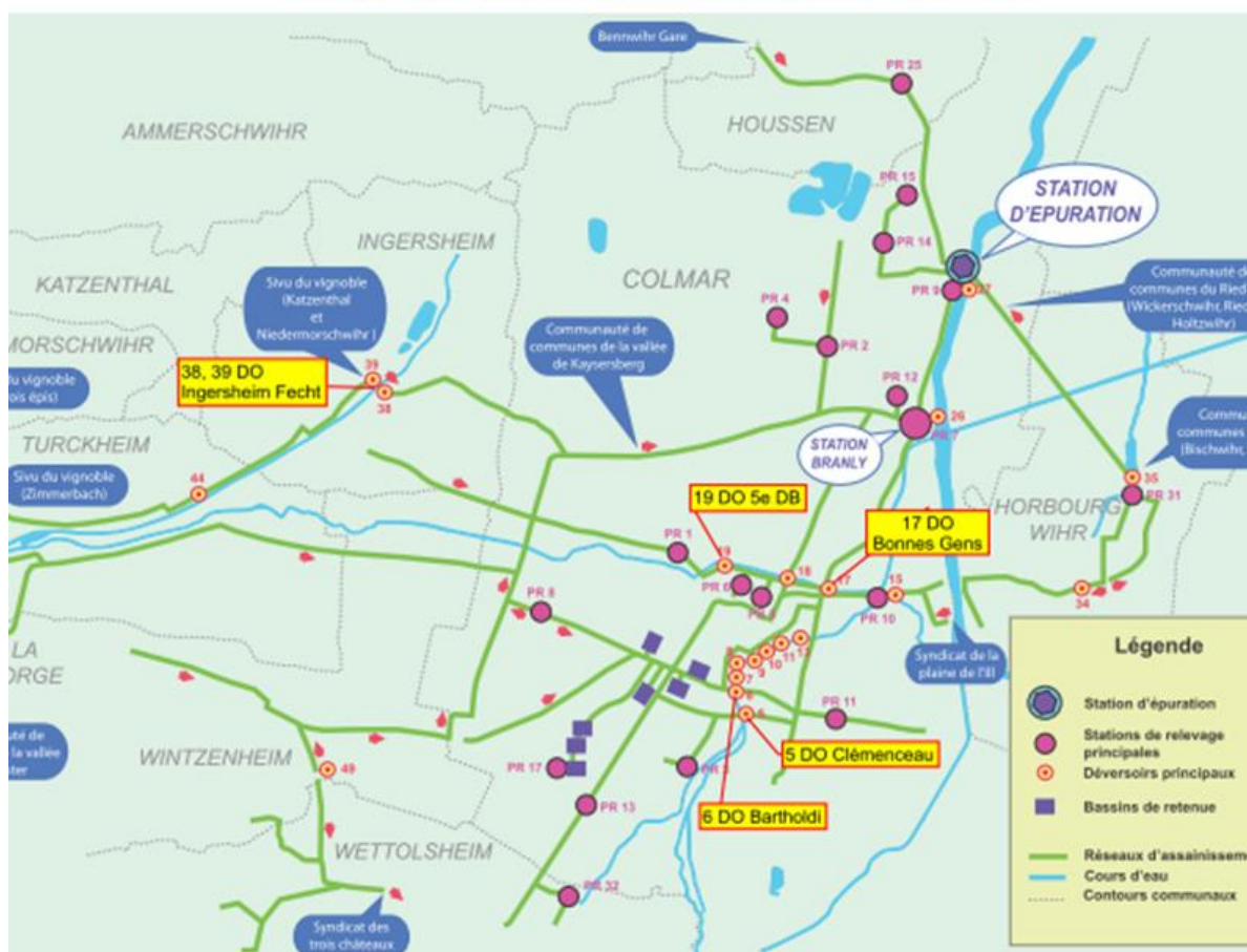
Schéma de principe de l'assainissement collectif – Source " Descriptif des dispositifs d'autosurveillance des déversoirs d'orage de la Colmar Agglomération »
